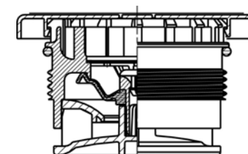
REF 010319 Bouchon M 2" dégazage/regazage pour couvercle Sch 010266
