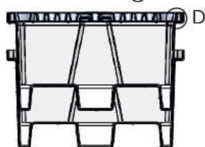
COUPE C-C
